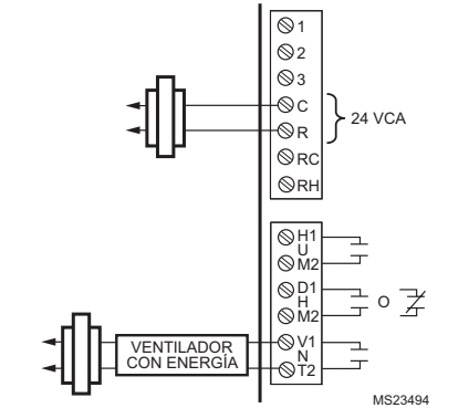
Conexión típica de deshumidificador con energía (deshumidificador de hogares).
