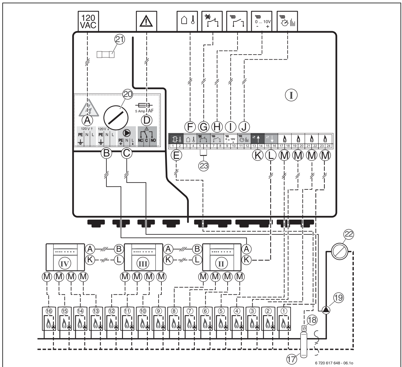
Fig. 12 Wiring diagram
