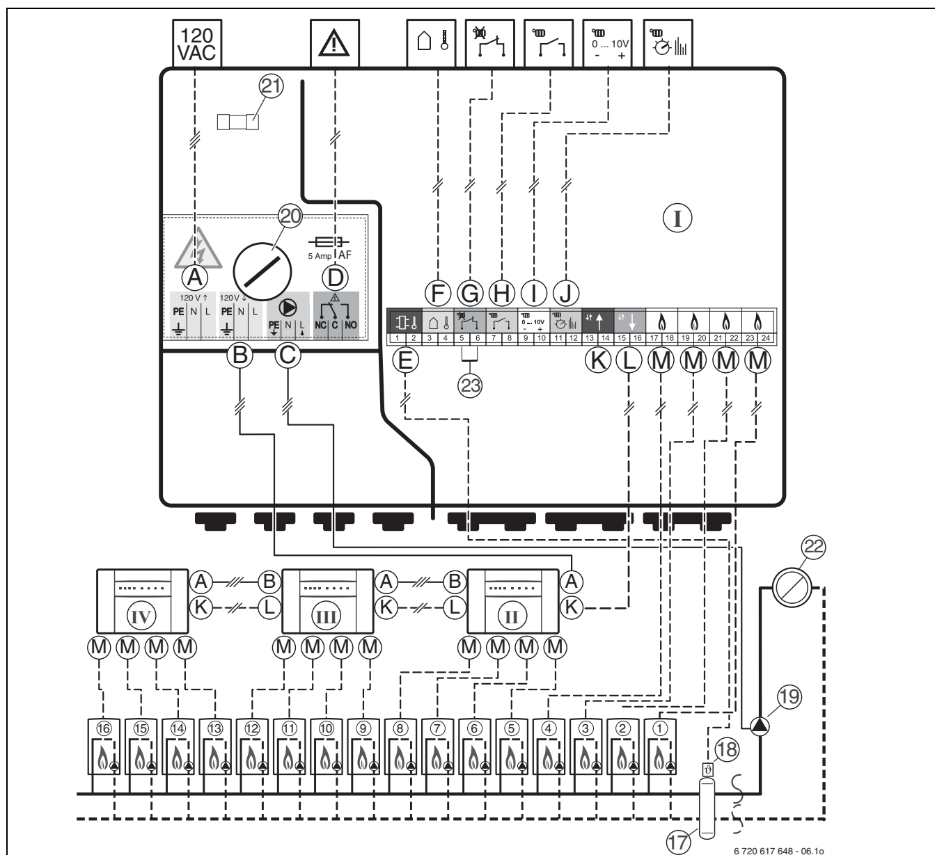
Fig. 24 Schéma de connexion
