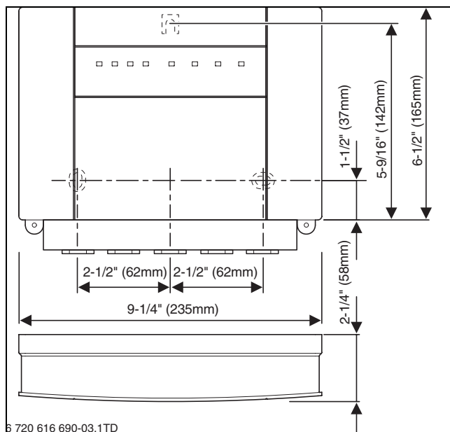
Fig. 2 Dimensions
