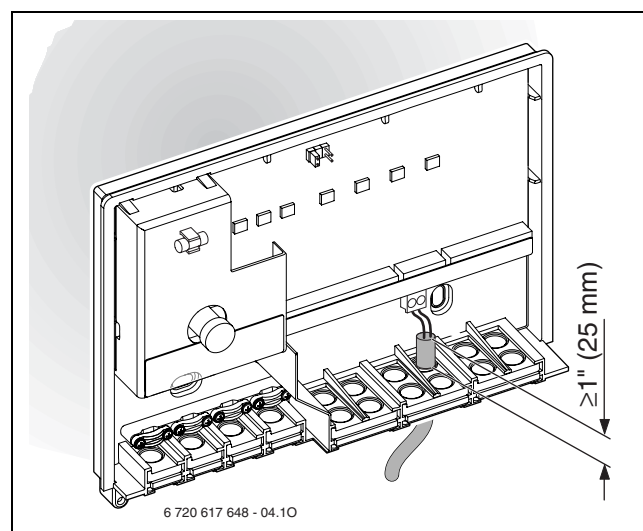
Fig. 21 Protection contre les projections d'eau
