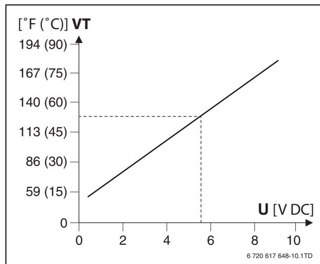
Fig. 17 Rapport entre la tension d'entrée et la température de départ
