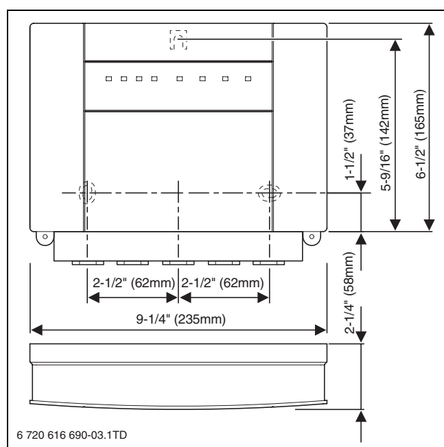
Fig. 14 Dimensions
