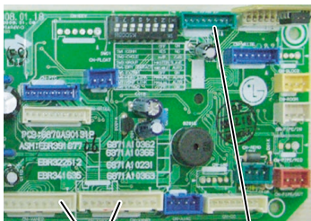
CN-VANE 1,2 CN-DISPLAY
