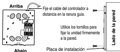
(parte frontal de la placa de instalación)
