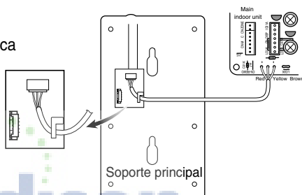
Fijación del mando a distancia
