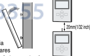
Fijación del mando a distancia
