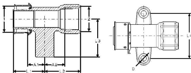
Viega PEX Press Fire Sprinkler Adapter
