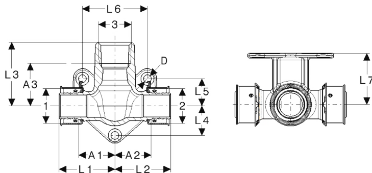
Viega PEX Press Fire Sprinkler Vertical Tees
