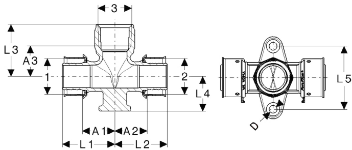
Viega PEX Press Fire Sprinkler Horizontal Tees
