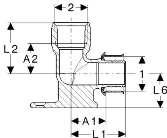
Viega PEX Press Fire Sprinkler Elbows
