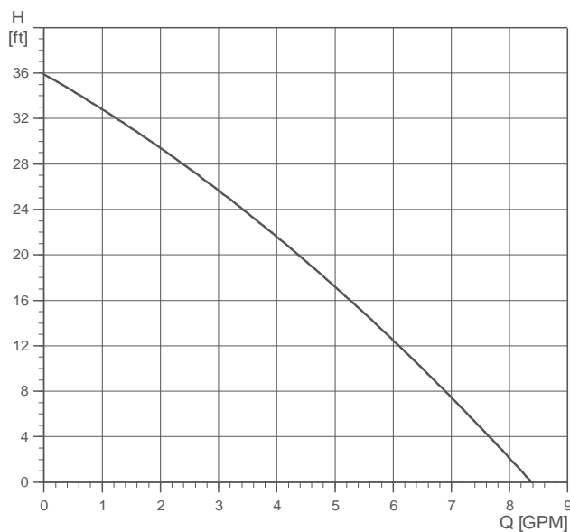
UP 15-100 F
