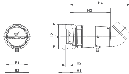
UP 10-16 B5/BN5
