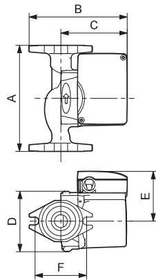
UP 15-10 FR
