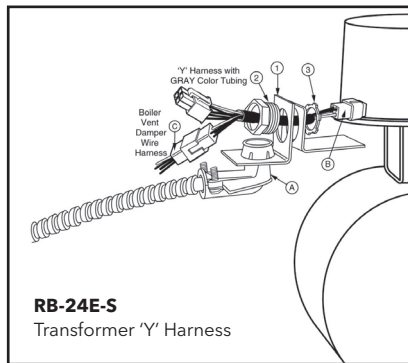
Wiring Diagrams
