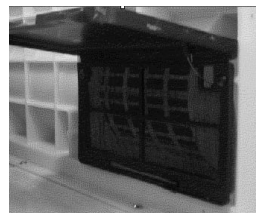
Ilustración B – Extracción del filtro de ventilación
